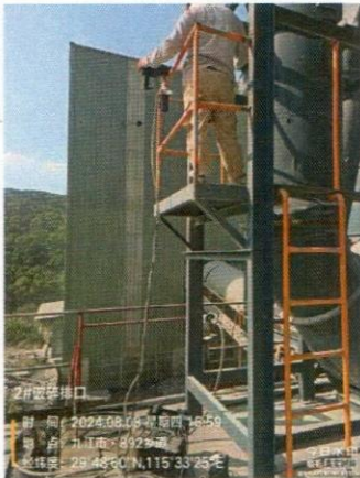
照片 17: 2#破碎机
